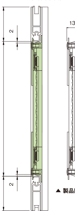
▲ 網戸枠への納まり図 (着色部=製品)
