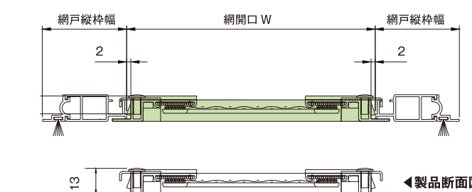
▲ 網戸枠への納まり図 (着色部=製品)
