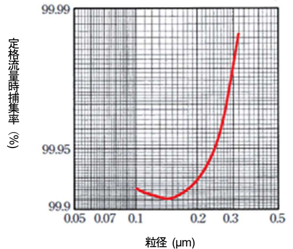
HEPA フィルター粒別捕集率
