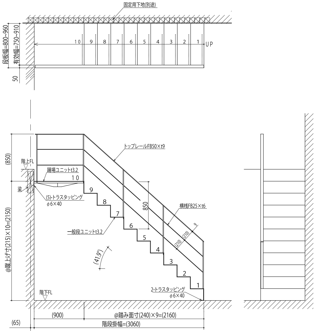
製品納まり図(横棧手すり)
