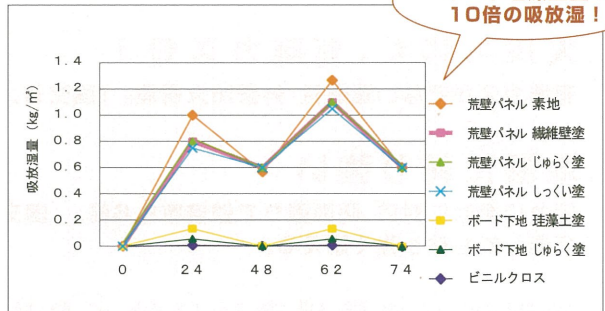
【図1】 吸放湿の繰り返し試験の比較
