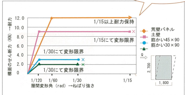
【図2】 復元力特性モデルの比較
