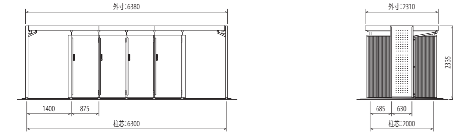
寸法図 (DCB-63-4B-1400F)
