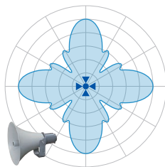
単体ホーンスピーカー (4方向設置時) 2kHz指向性イメージ
