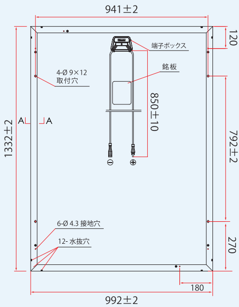
背面図
