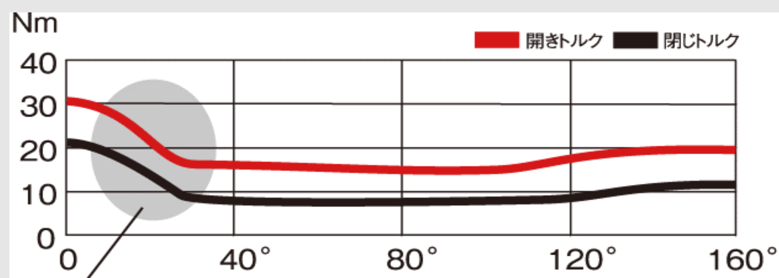
DORMAスライドチャンネル式 ハートカム式ドアクローザ
