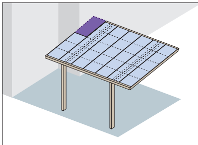
前枠側：間口台形納まり
