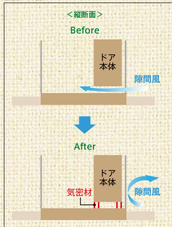
室内ドア納まり※1
