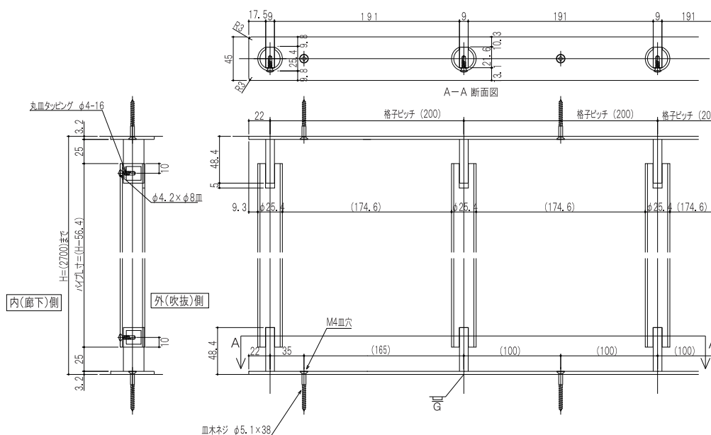
製品納まり図 丸パイプの場合
