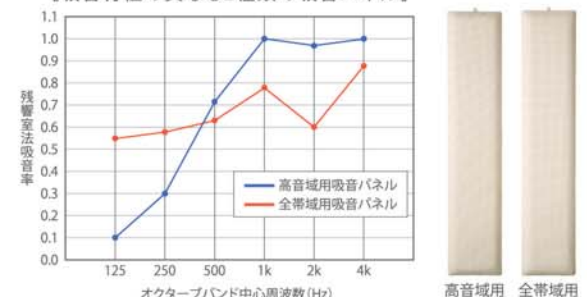
【吸音特性の異なる2種類の吸音パネル】
